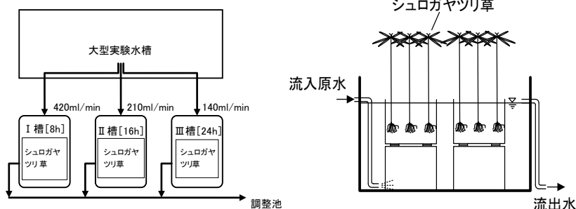
図-1 実験装置
